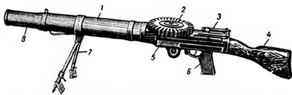
Рис. 140. Общий вид пулемёта Льюиса обр. 1915 г.: 1 — кожух; 2 — магазин; 3 — привод; 4 — прицел; 5 — ствольная коробка; 6 — рукоятка управления огнём; 7 — сошка; 8 — лотрубок
