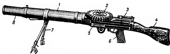
Рис. 140. Общий вид пулемёта Льюиса обр. 1915 г.: 1 — кожух; 2 — магазин; 3 — прицел; 4 — приклад; 5 — стальная коробка; 6 — рукоятка управления огнём; 7 — сошка; 8 — патробо́к
