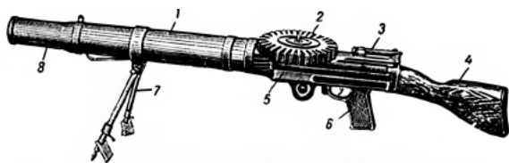
Рис. 140. Общий вид пулемёта Льюиса обр. 1915 г.: 1 — кожух; 2 — магазин; 3 — прицел; 4 — приклад; 5 — ствольная коробка; 6 — рукоятка управления огнём; 7 — сошка; 8 — лотушок
